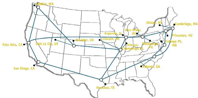
NSFNet, 1992
